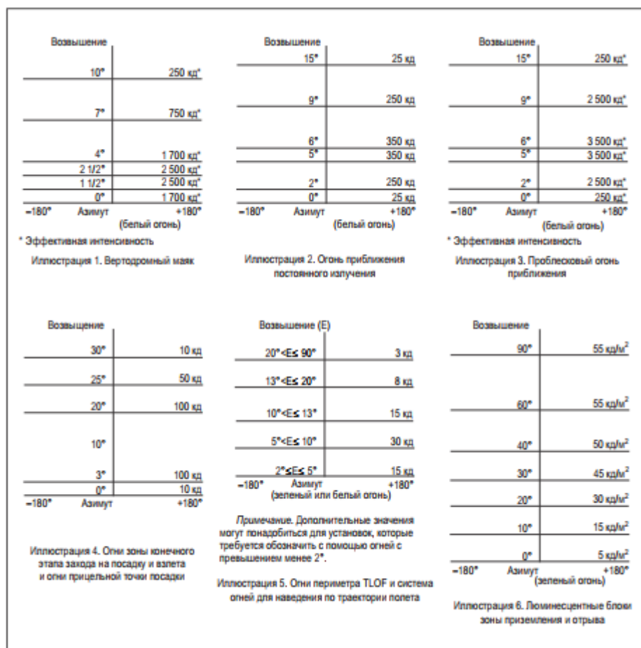
Рис. 5-12. Диаграммы изокандел
