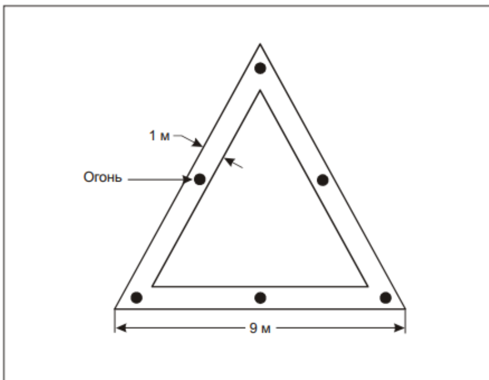
Рис. 5-7. Маркировка прицельной точки посадки
