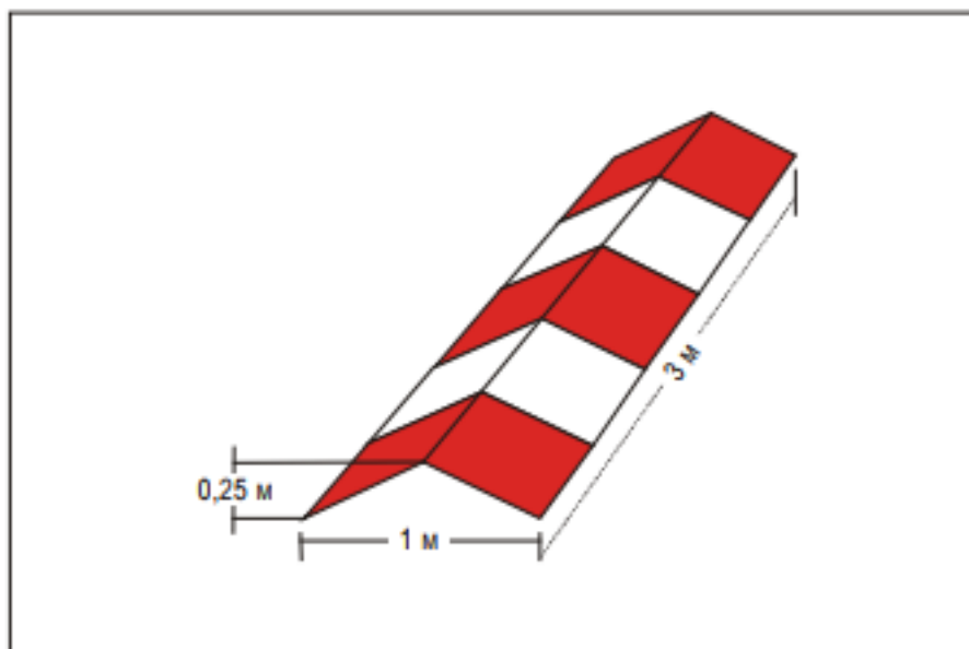
Рис. 5-6. Маркер границы зоны FATO типа ВПП
