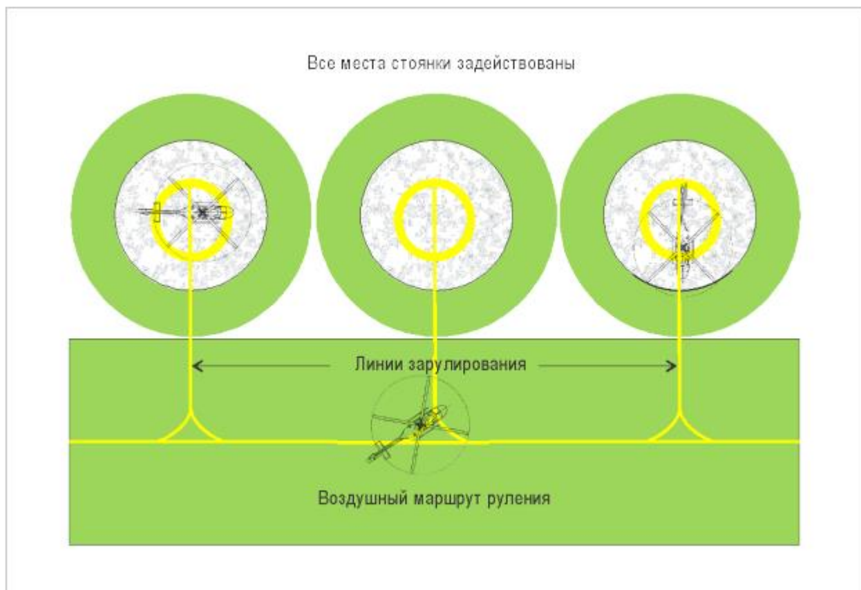
Рис. 3-5. Места стоянки, предназначенные для выполнения разворотов (с воздушными маршрутами руления) : одновременное использование
