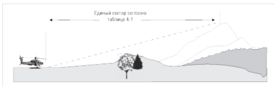
в) Поверхности захода на посадку и набора высоты при взлете, наклонный профиль "С": градиент 12,5 %
