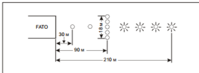
Рис. 5-13. Система огней приближения
