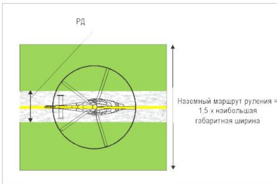
Рис. 3-3. РД/наземный маршрут руления для вертолетов
