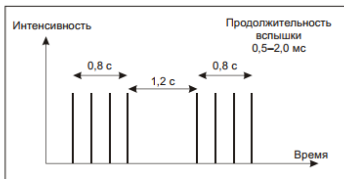
Рис. 5-11. Характеристики вспышки вертодромного маяка
