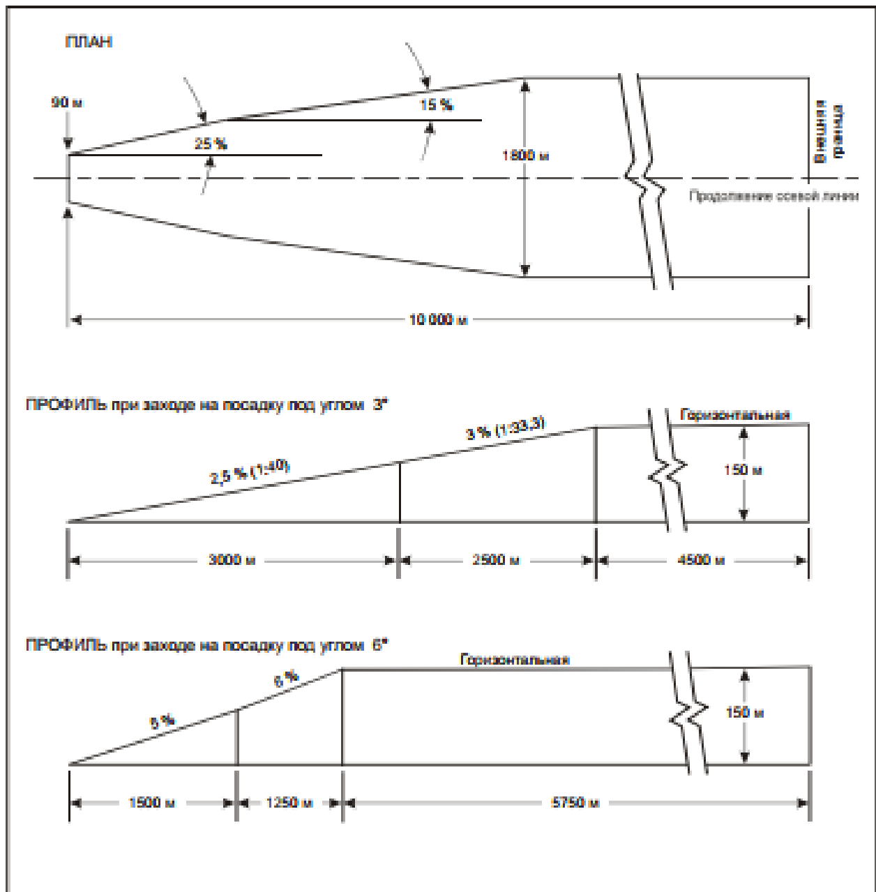
Рис. А-3. Поверхность захода на посадку для FATO, оборудованной для точного захода на посадку
