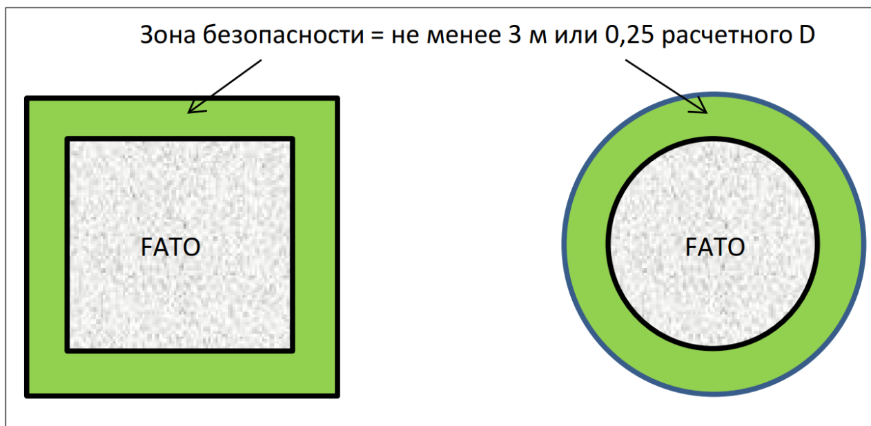
Рис. 3-1. FATO и связанная с ней зона безопасности
