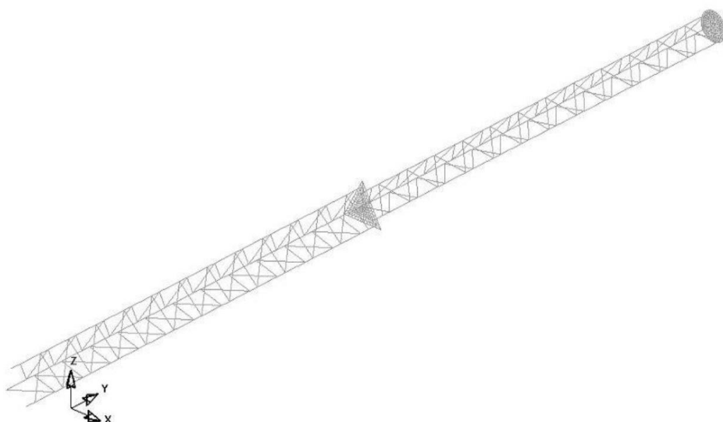
б) опора огней приближения: алюминиевая решетчатая конструкция
