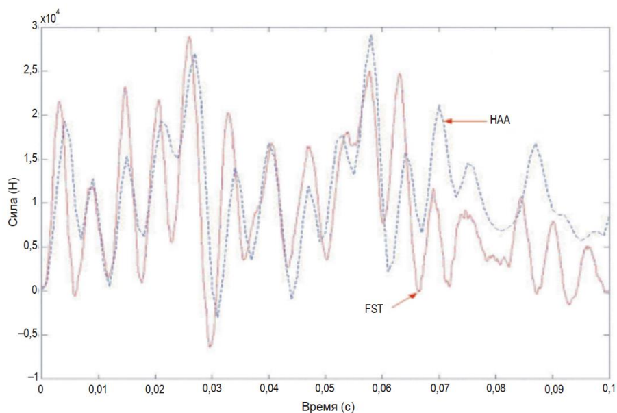
Рисунок 6-7. Ударные силы, рассчитанные с использованием подхода методом гибридного анализа (HAA), в сравнении с результатами натурного испытания (FST)
