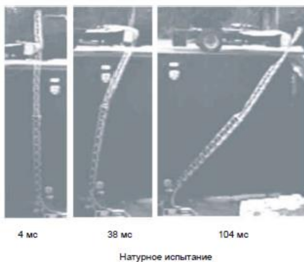
Рис. 6-3. События удара по данным моделирования в анализе методом конечных элементов (FEA) и натурного испытания: скорость соударения 140 км/ч; удар в верхнюю часть; масса верхней части 5,44 кг; жесткий ударный механизм
