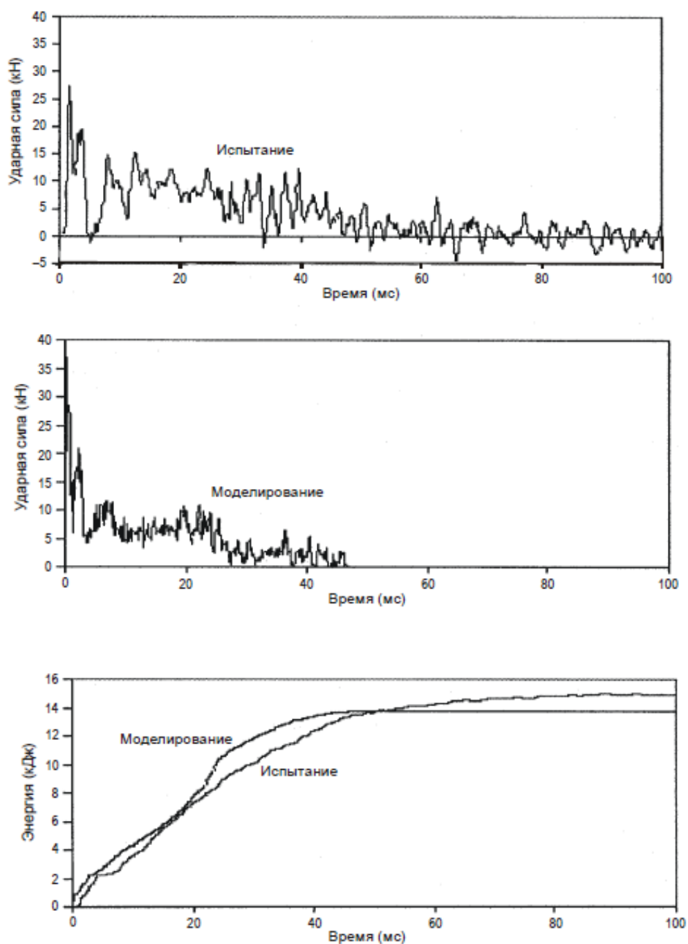
Рис. 6-4. Ударная сила и энергия: скорость соударения 140 км/ч; удар в бок; жесткий ударный механизм
