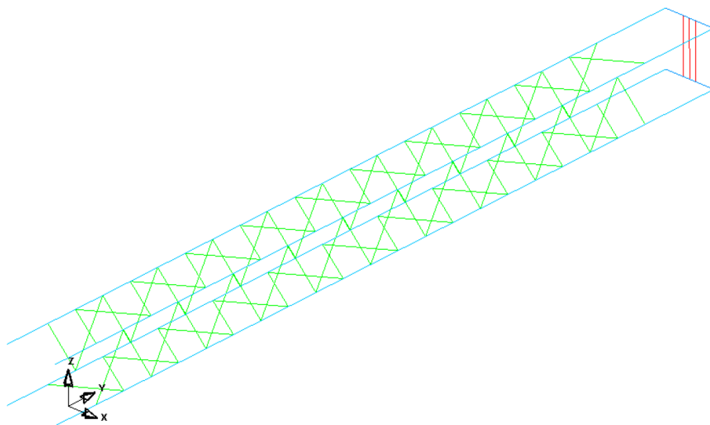
а) опора огней приближения: стеклопластиковая решетчатая конструкция
