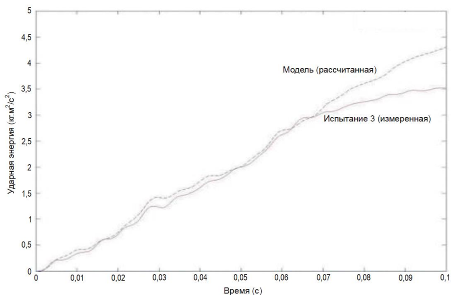
Рисунок 6-8. Ударная энергия, рассчитанная с использованием подхода методом гибридного анализа, в сравнении с результатами натурного испытания.
